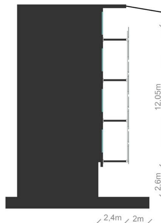
CORTE EDIFICIO INACAP
