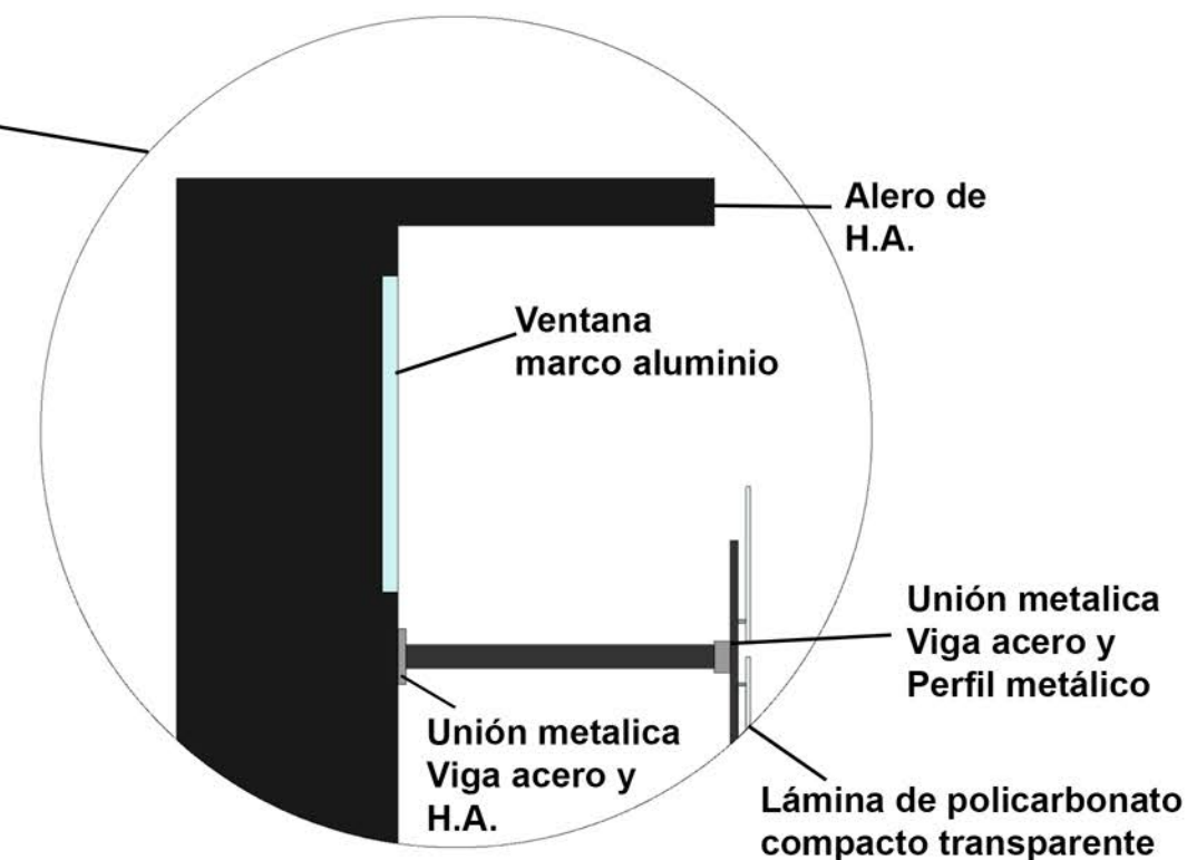
DETALLE CONSTRUCTIVO
