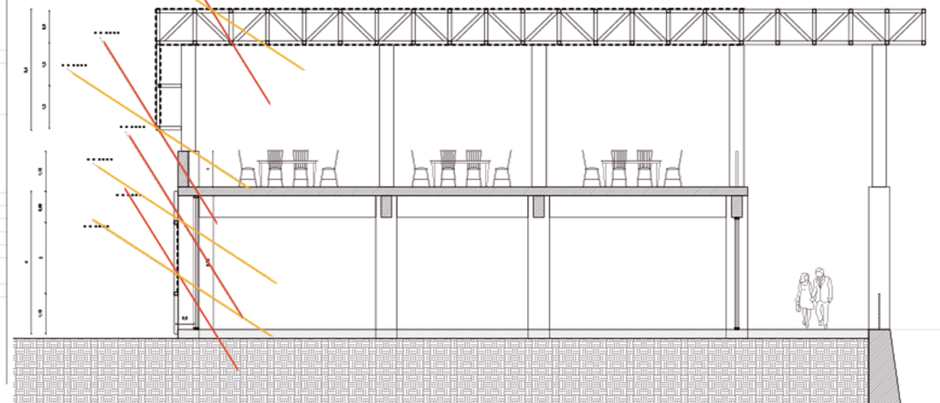
CORTE TRANSVERSAL TERRAZA RESTORANT CORTE B-B'
