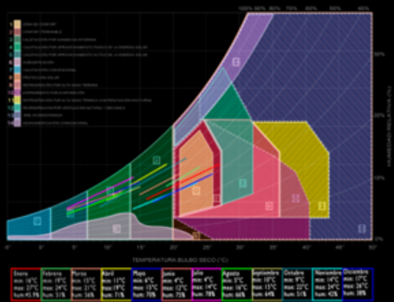
Grafico de Givoni
