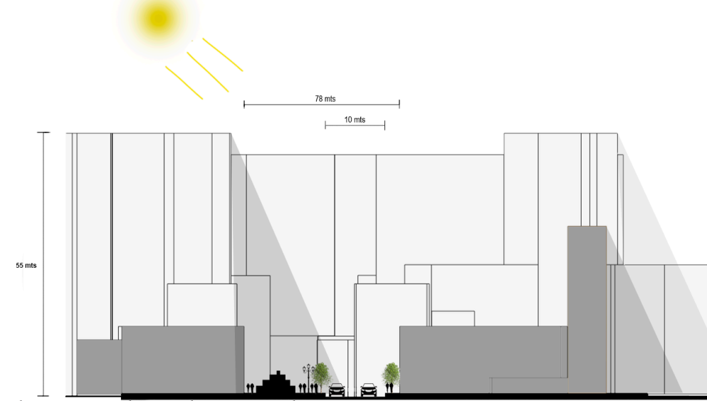
Plaza Bernardo Leighton - Escala 1:100
